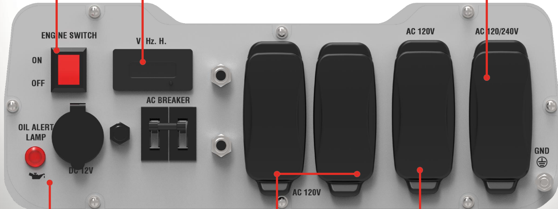
(1) 120V AC 30A L5-30R
